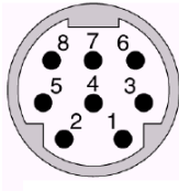
8 针圆形母座管脚图
