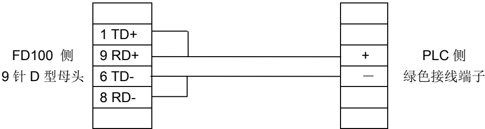
MD2-Emerson-RS485 (PORT1) 电缆连线图
