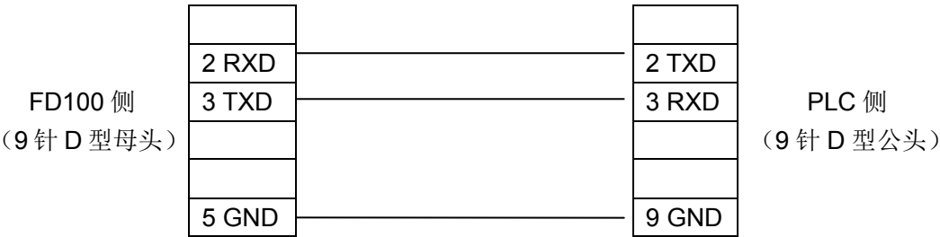
MD2-CQM 电缆连线图
