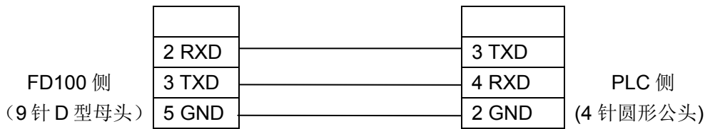
MD2-FATEK FBS 系列电缆连线图
