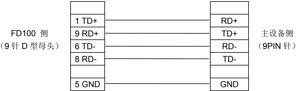
MD2-MODBUS-RS422 连线图
