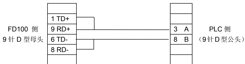
MD2-S7-200 电缆连线图
