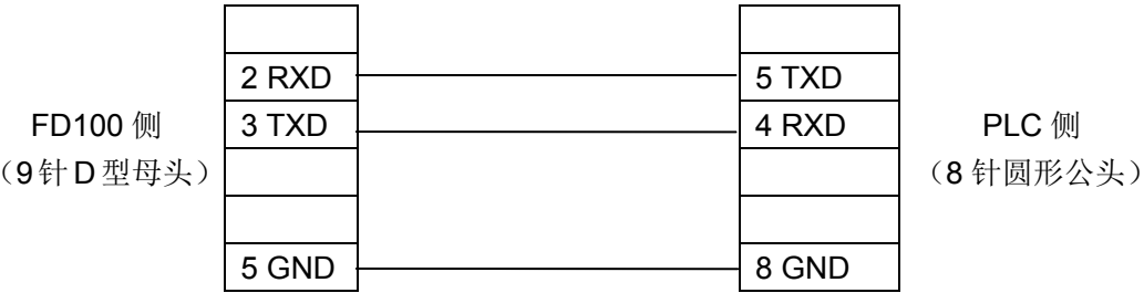
MD2-DVP 电缆连线图
