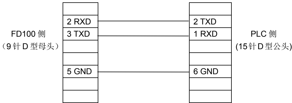
MD2-FATEK FBS 系列电缆连线图
