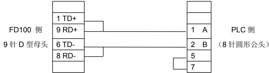
MD2-TWIDO 电缆连线图
