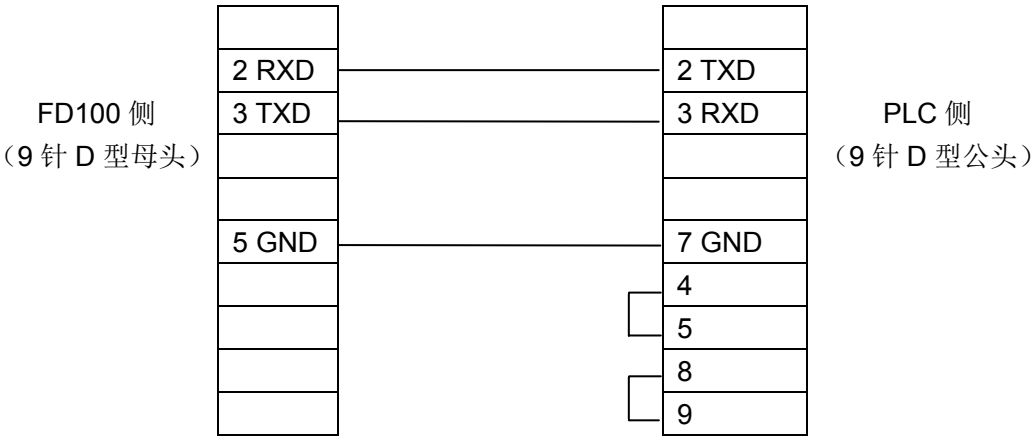
MD2-FP 电缆连线图
