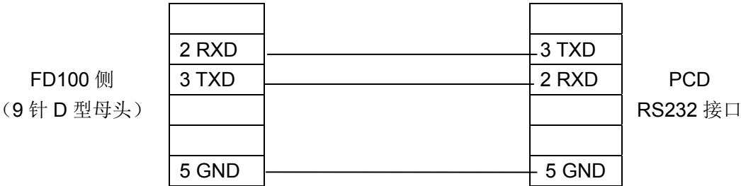
MD2-SAIA-RS232 连线图
