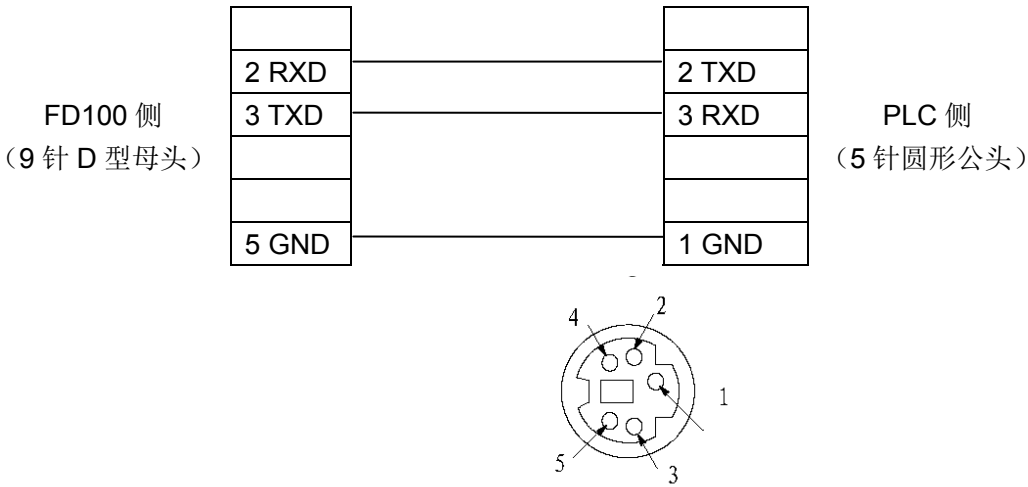
松下 5 针圆形母座管脚图
